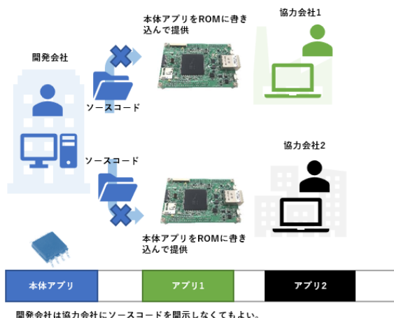
図 1-2. ソースコード無しで開発を分担
