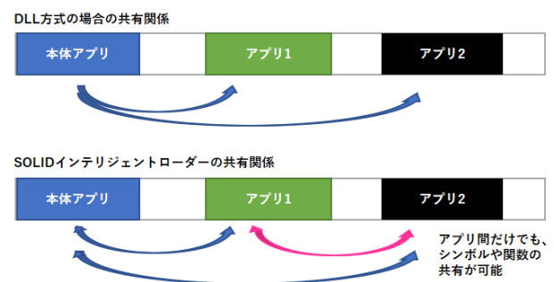
図 3-4 相互参照の関係の相違
