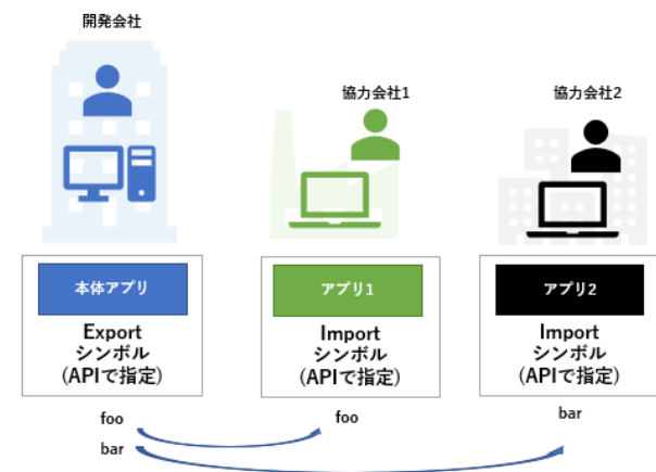
図 2-2. 本体アプリのシンボルをサブアプリで共有する (API を利用)
