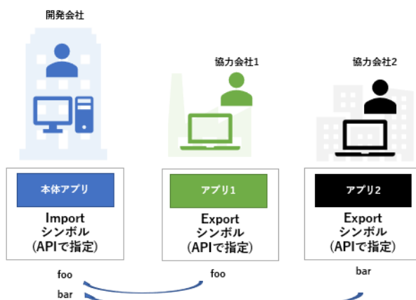
図 2-4 サブアプリのシンボルを本体アプリで共有する (API を利用)
