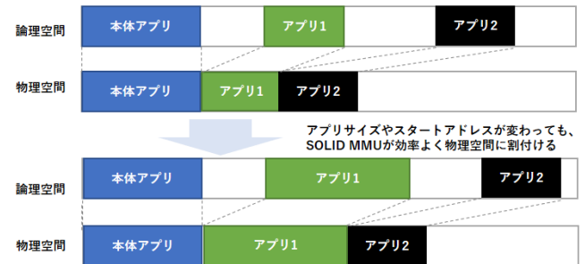
図 3-7 ロードが物理空間に効率よく実行モジュールを配置
